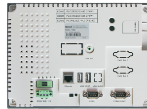
背面图
