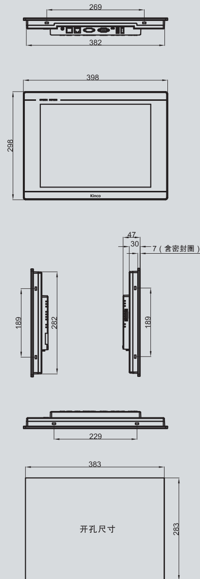
尺寸图 (单位: mm)
